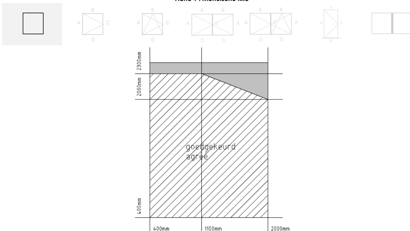
Performance de la fenêtre cf. NBN EN 14351-1
