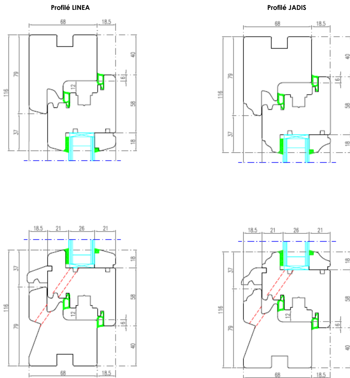
Fig. 1: Types de profilés pour fenêtre (coupe verticale)
