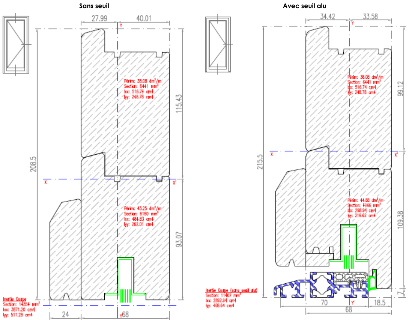
Fig. 2: Bas de porte (coupe verticale)
