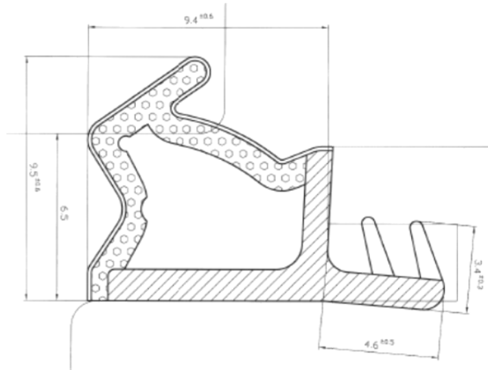
Fig. 6: Joints d'étanchéité et de frappe
