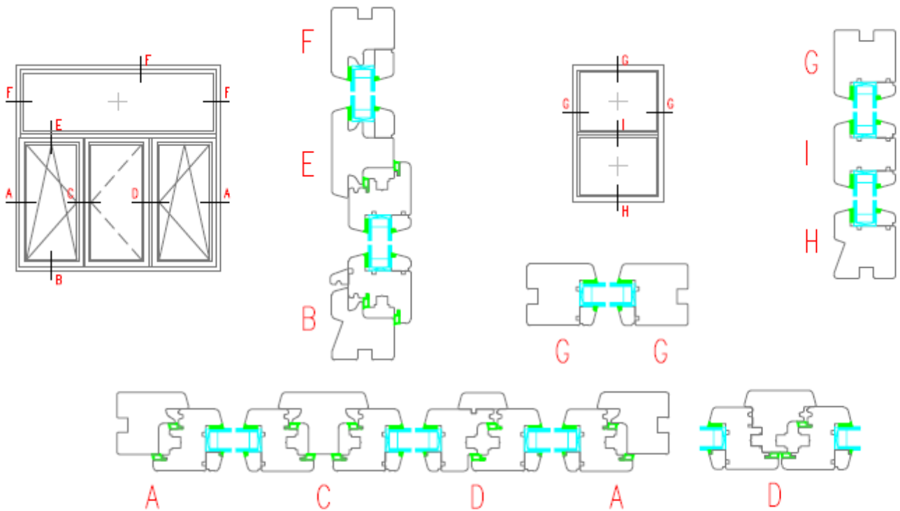
Fig. 3: Géométrie des fenêtres
