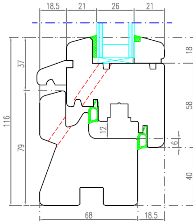
Fig. 5: Orifices de drainage et d'aération (coupe verticale - traverse basse)
